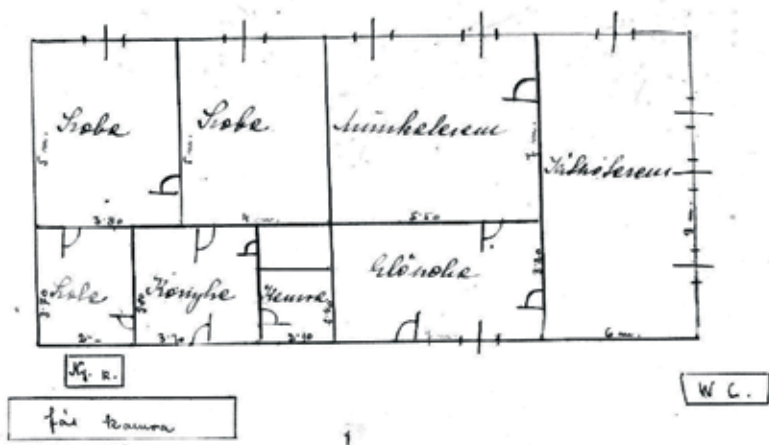
13. A kétegyházi Szent Imre utca 25. sz. alatti kisdóvoda épület vázlata
