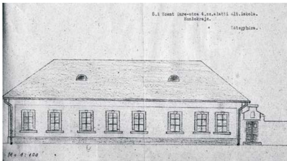
14. A Szent Imre utca 4. szám alatti általános iskola homlokrajza (Fiú iskola)
